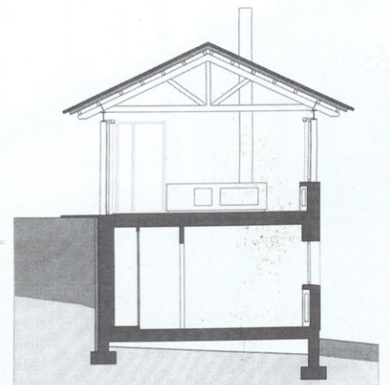
12 · SECCIÓN TRANSVERSAL
